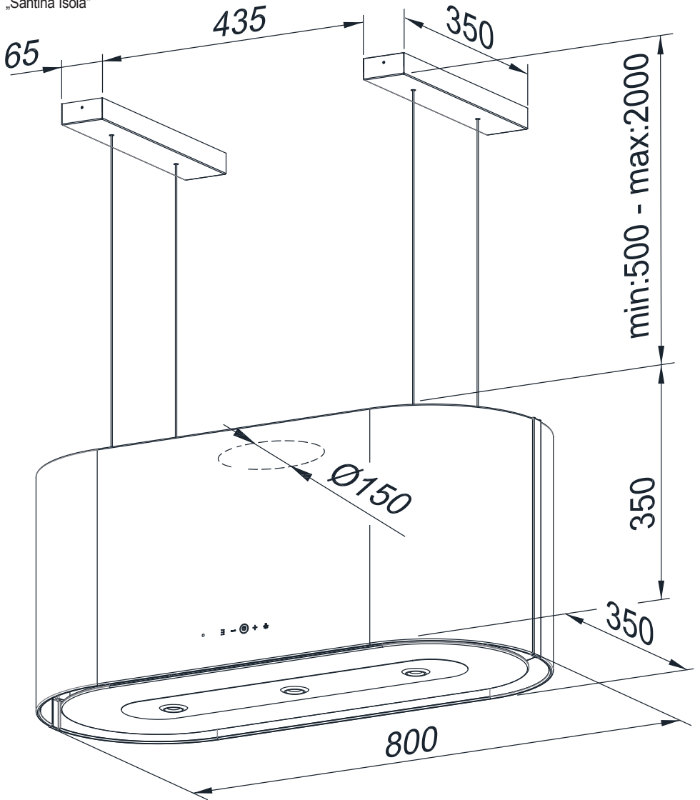
Abb. 17 Abmessungen Modell „Santina Isola“
